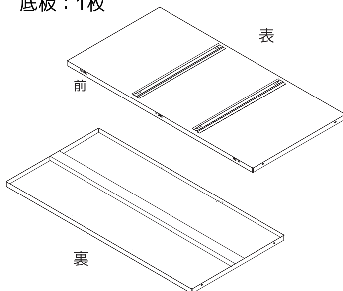
底板：1枚
