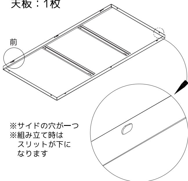
天板：1枚
