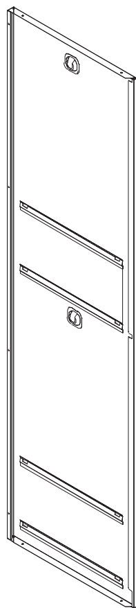
右側板：1枚
