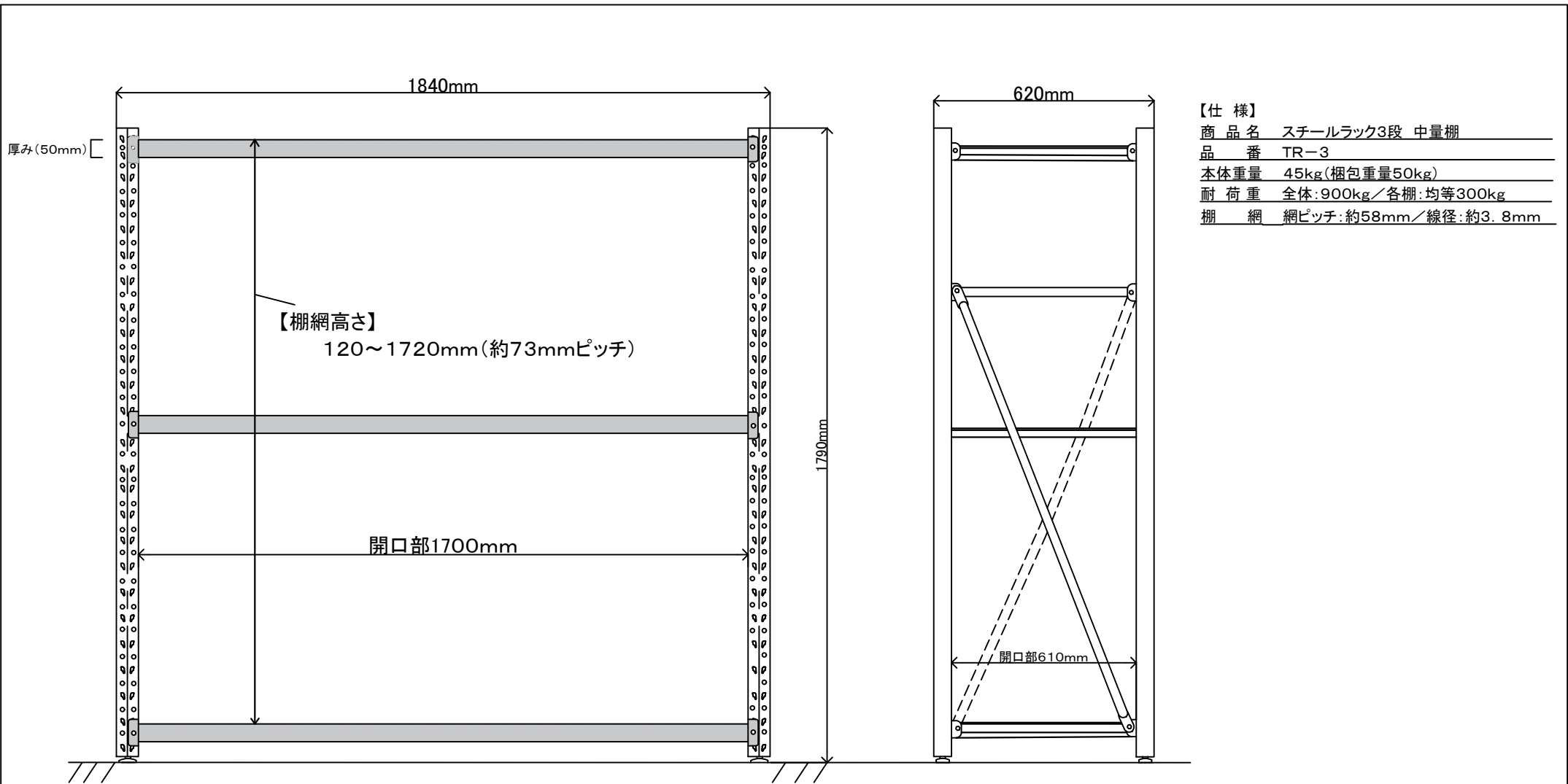
(正面図)
